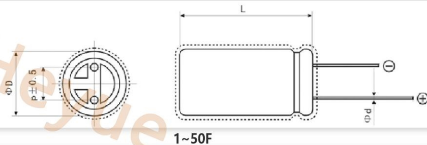
产品图纸
