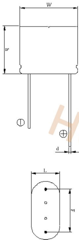
产品图纸
